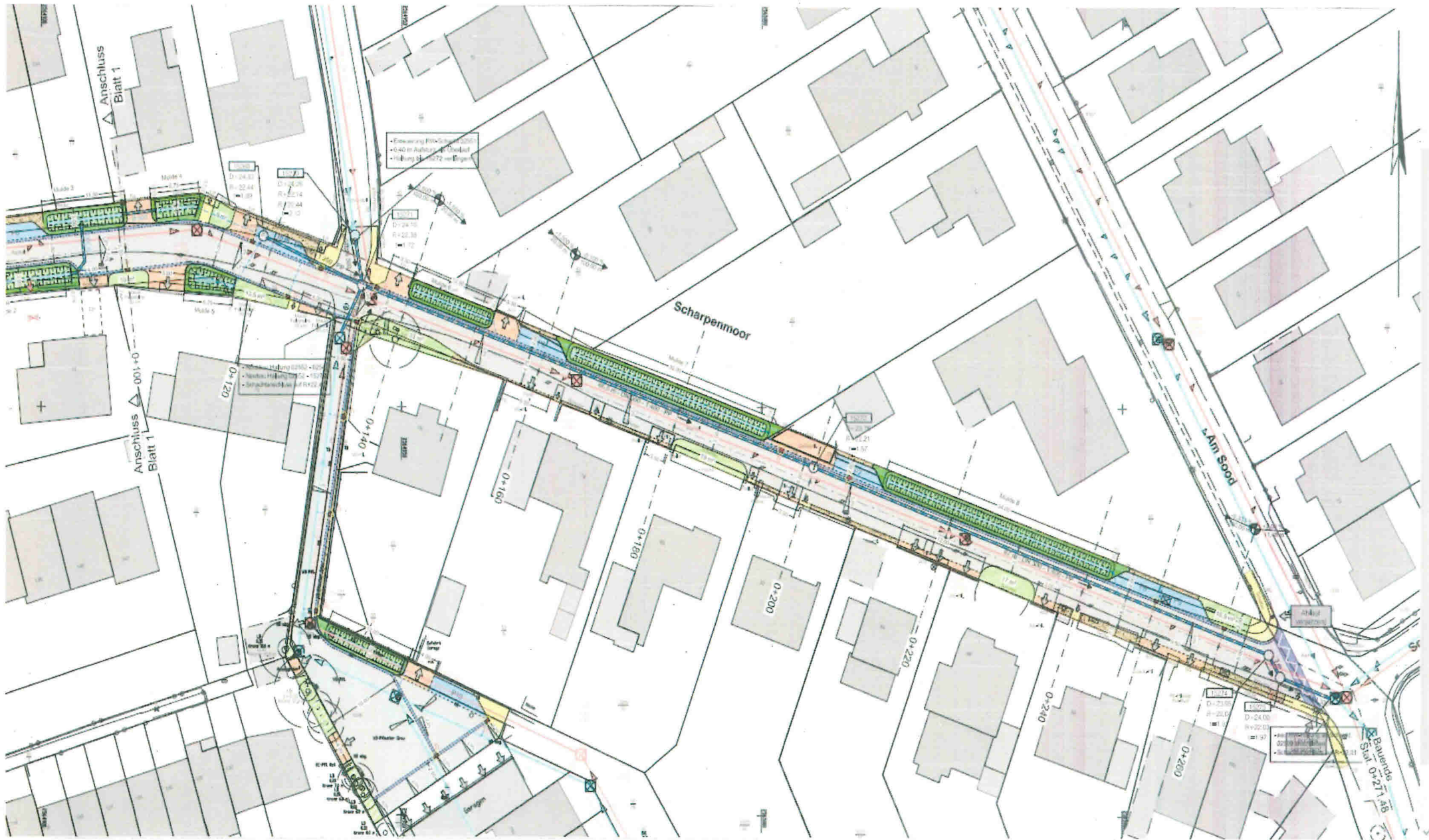
Variante 2 (Mischverkehrsfläche)
