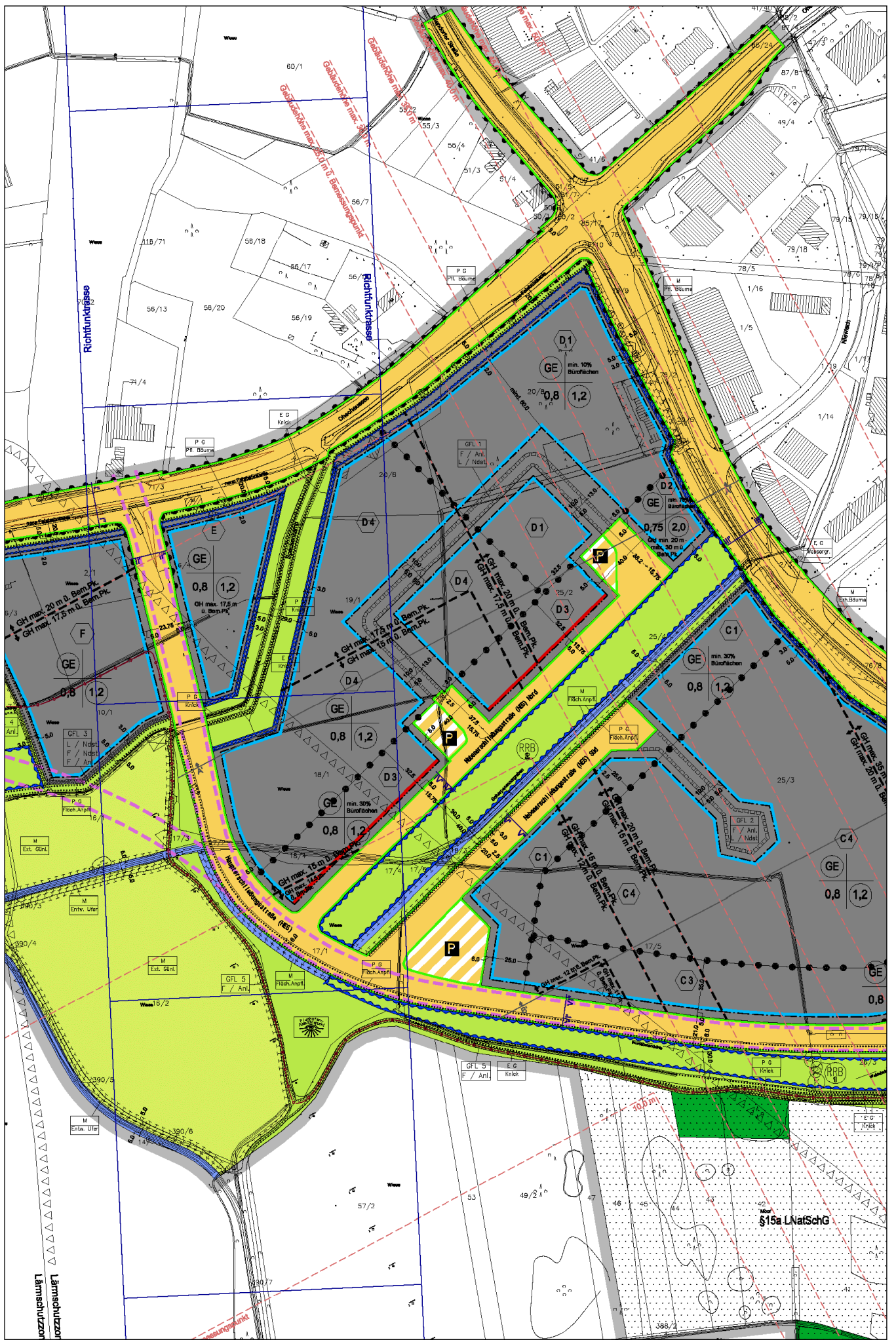
Anlage 4: zur Vorlage Nr. B 19/0718 des StUV am 05.12.2019 Hier: Planzeichnung des rechtskräftigen Bebauungsplanes Nr. 245
