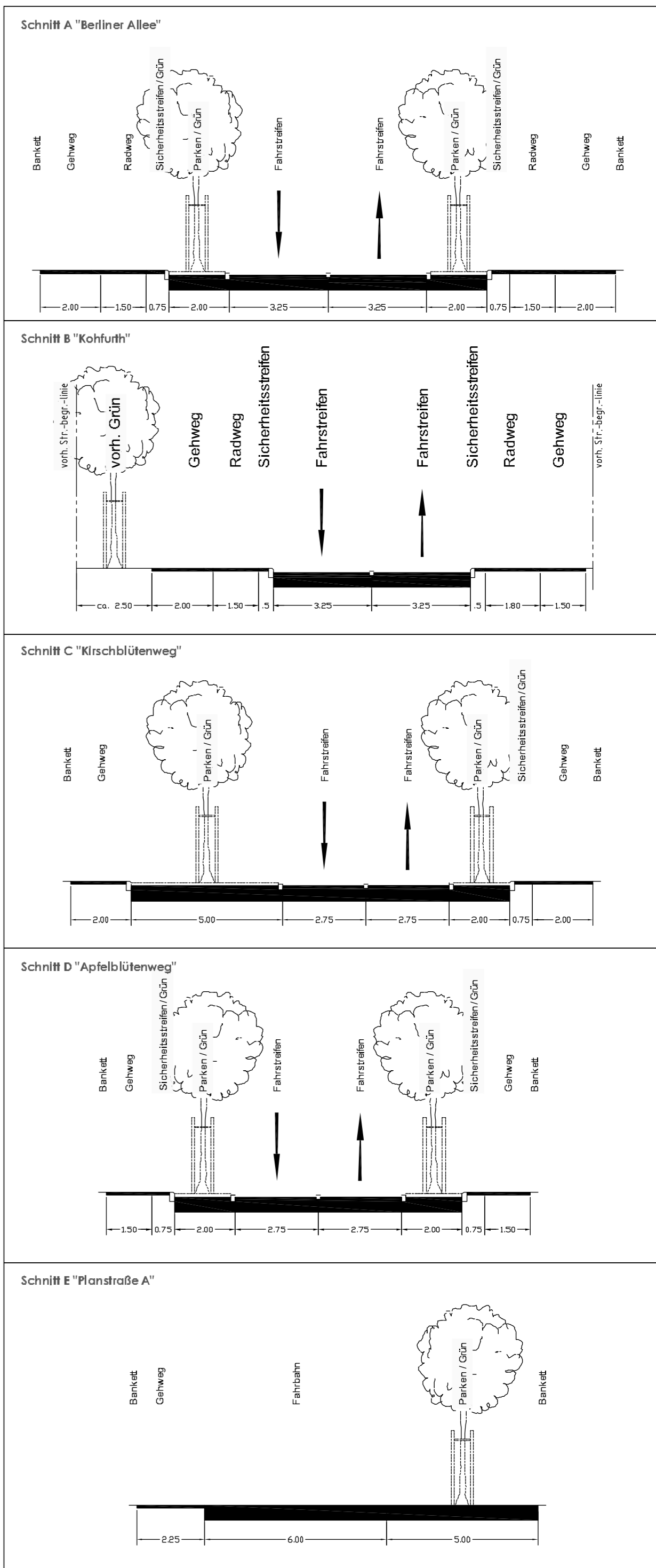
Straßenquerschnitte Darstellungen ohne Normcharakter M 1:150
