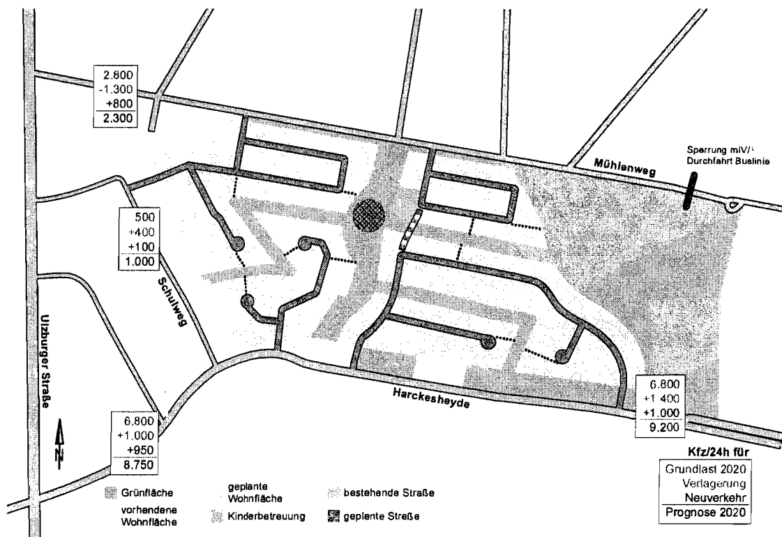
Grafik 7: Tagesverkehrsstärken an ausgewählten Querschnitten in Variante 1
