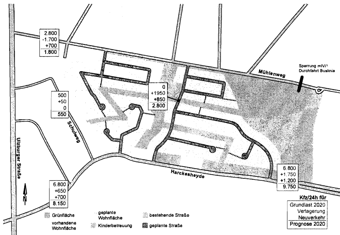
Grafik 10: Tagesverkehr an ausgewählten Querschnitten in Variante 4
