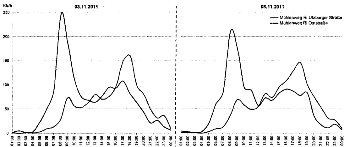
Grafik 3: Tagesganglinien der Verkehrsstärken im Mühlenweg
