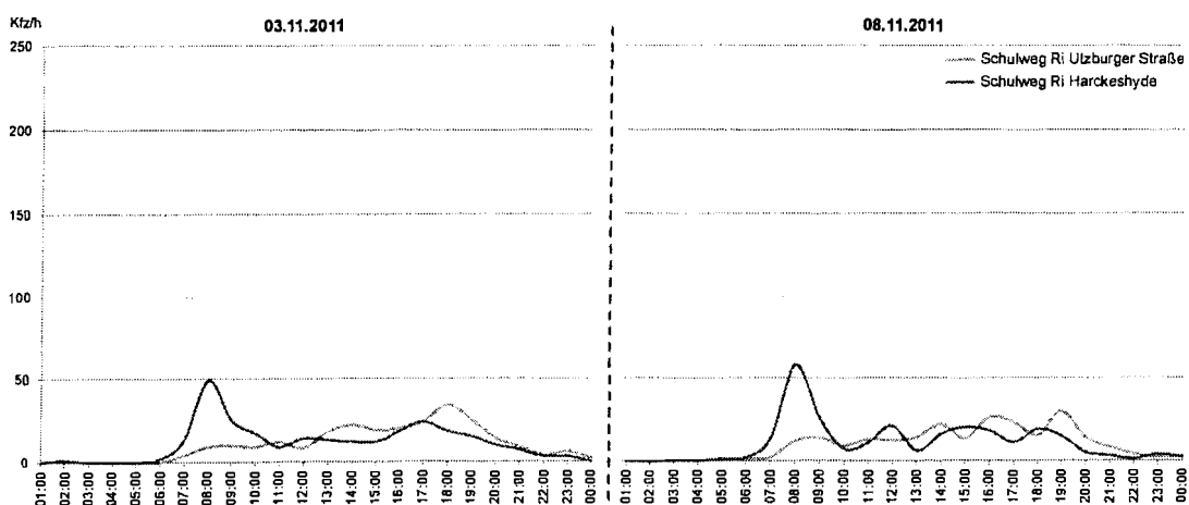
Grafik 4: Tagesganglinien der Verkehrsstärken im Schulweg
