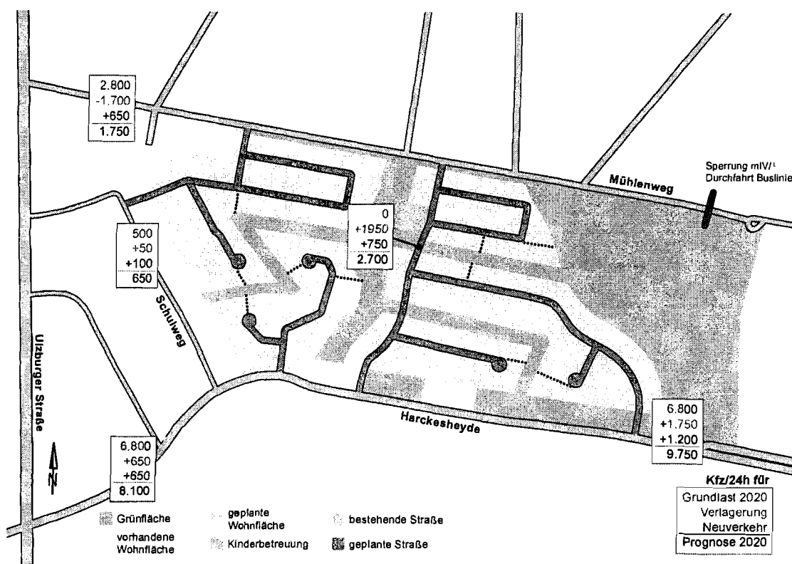
Grafik 9: Tagesverkehr an ausgewählten Querschnitten in Variante 3
