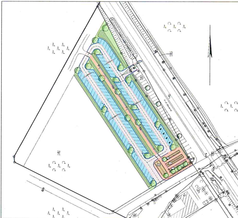
Planausschnitt des Lageplans für die Erweiterungsmaßnahme
