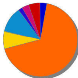
Ertragsaufspaltung Kreisdiagramm
