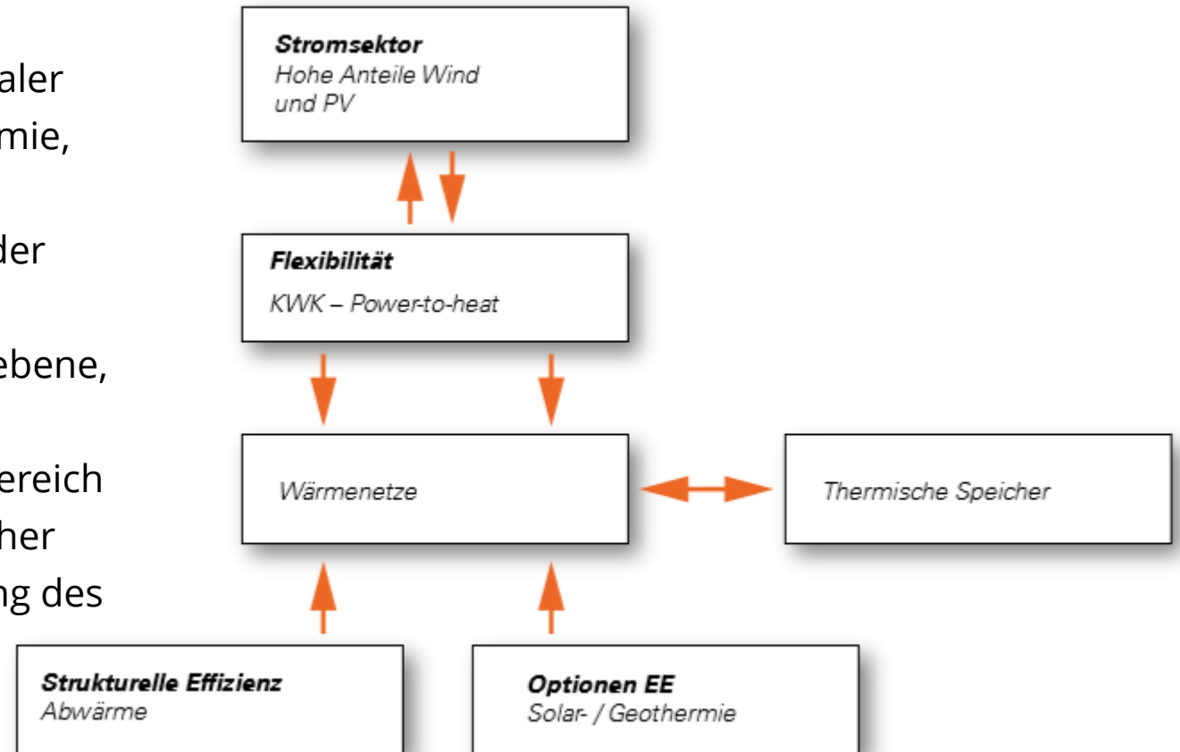
Abbildung 4: Gesamtübersicht über die stromnetzdienlichen Systemdienstleistungen von Wärmenetzen im Energiesystem mit sehr hohen Anteilen erneuerbarer Energien.
