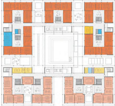
FUNKTIONSBEREICHE 2. OG
