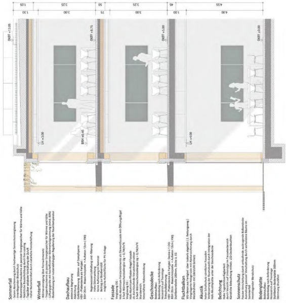
FASADENSICHT M 1:50
