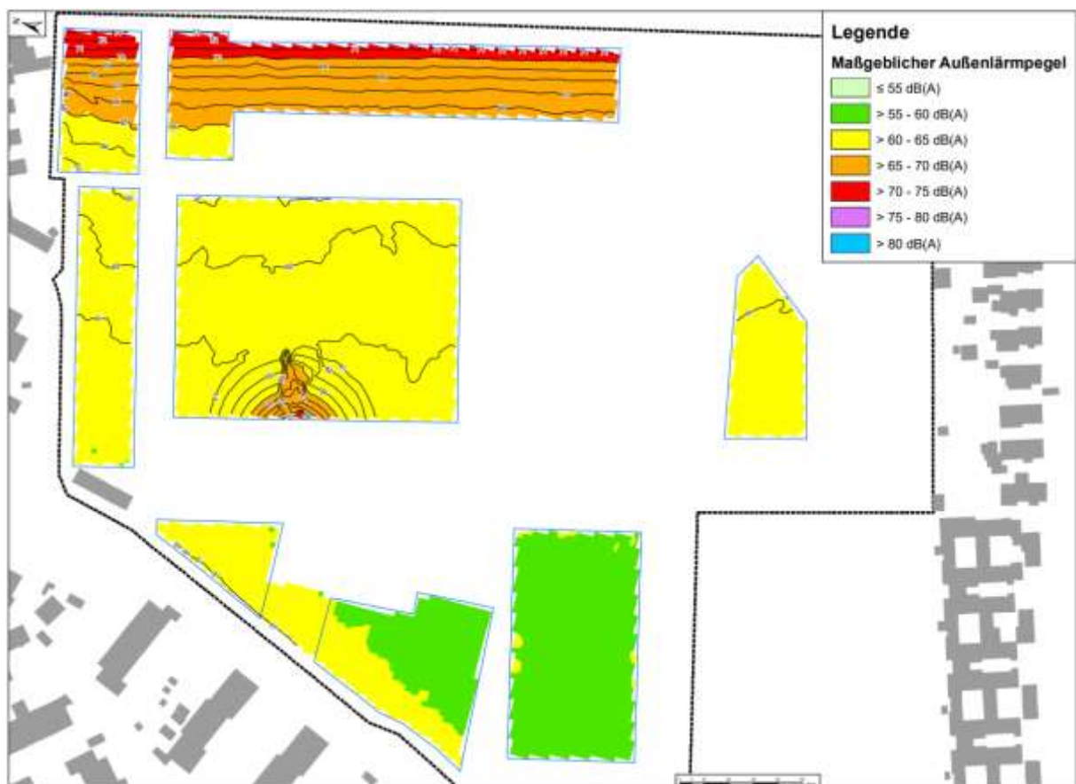
Nebenzeichnung 1
